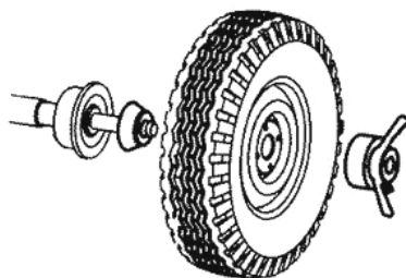
Рисунок 6.5 – Установка колеса
